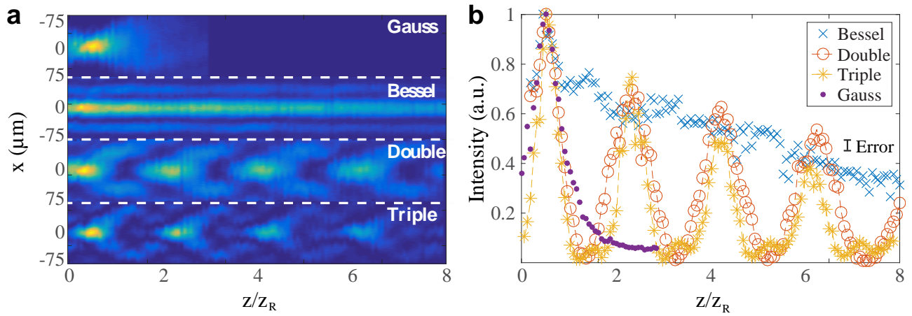
La propagazione di un normale fascio di luce (Gauss) soggetto a divergenza, e tre diversi fasci non-diffrattivi nella forma di fasci di Bessel beams e light droplets in diverse forme.
